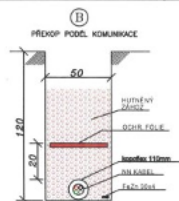
ŘEZY ULOŽENÍ KABELŮ NN-0,4kV
